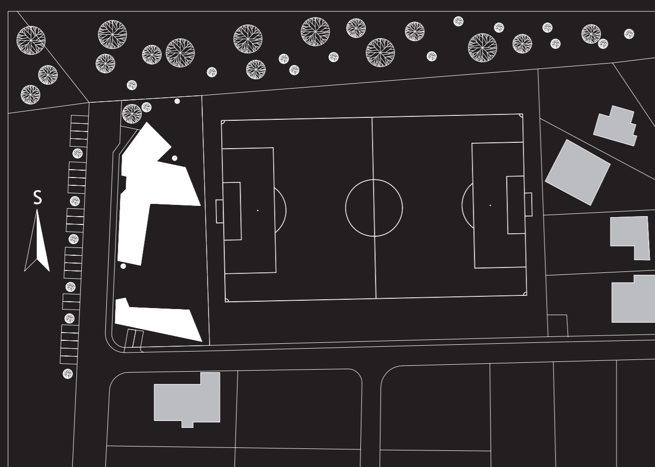
SITUACE M 1:1000
