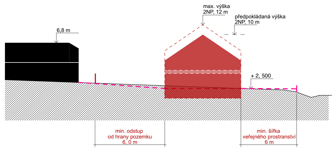
řez příčný - škola, sever
