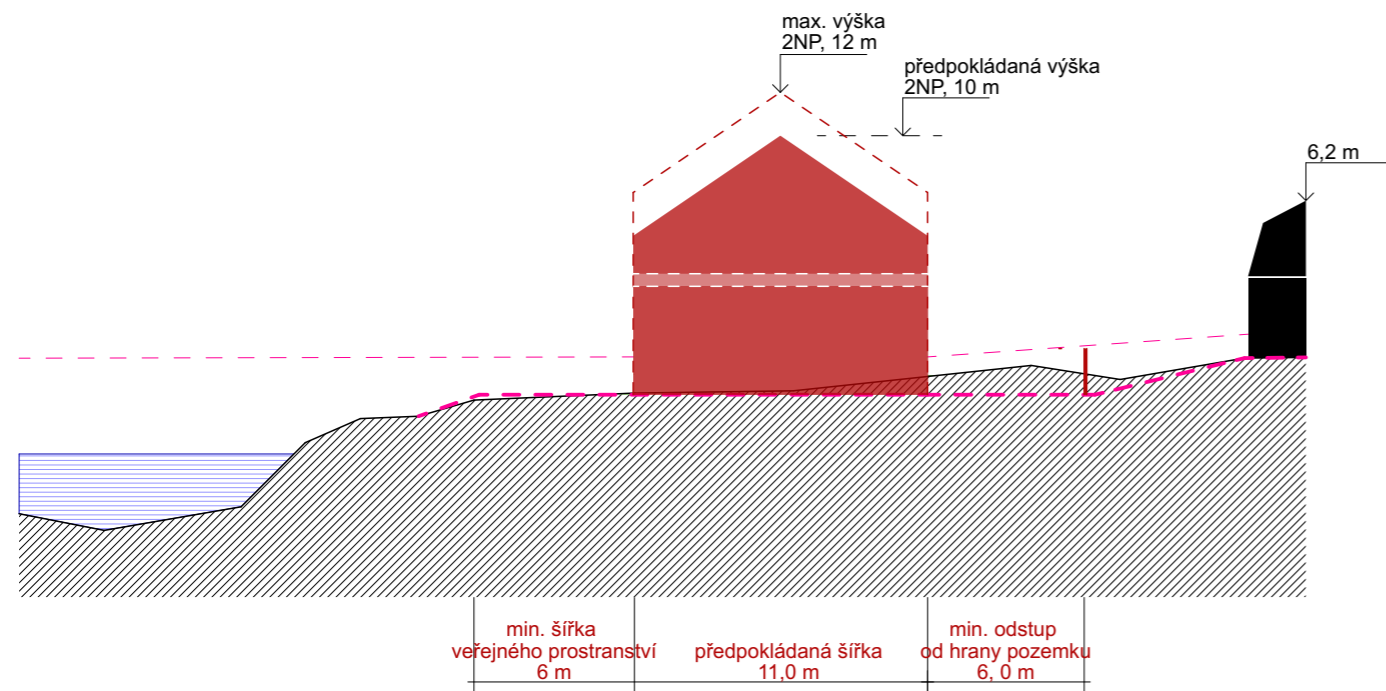
řez příčný - škola, jih
