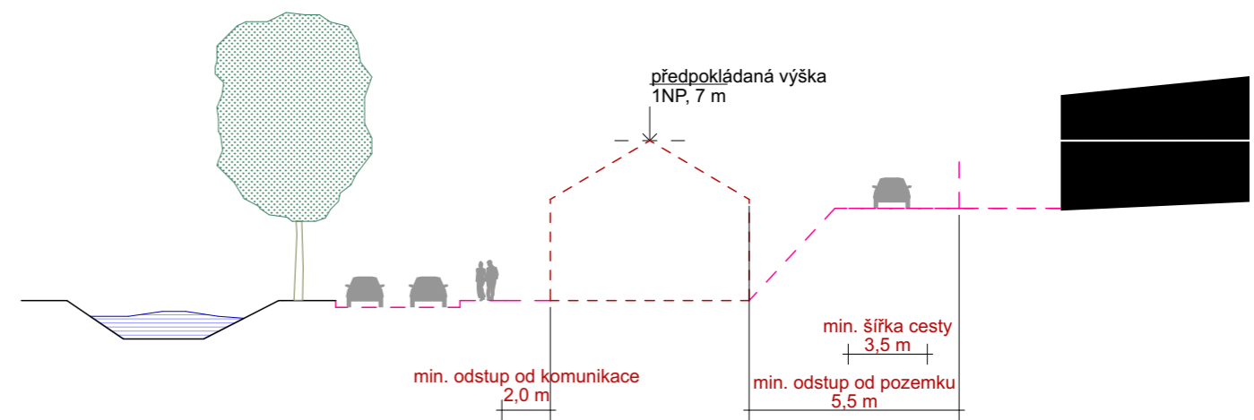
řez příčný - tělocvična
