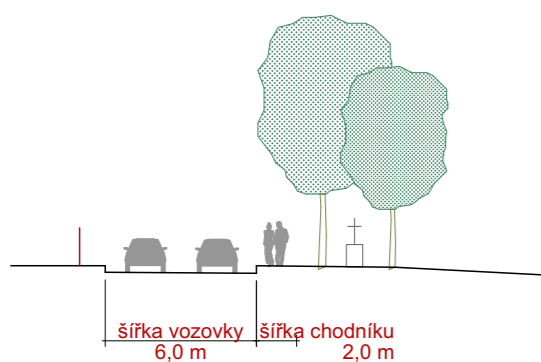
řez silnicí III/10176 - Starobabická stav
