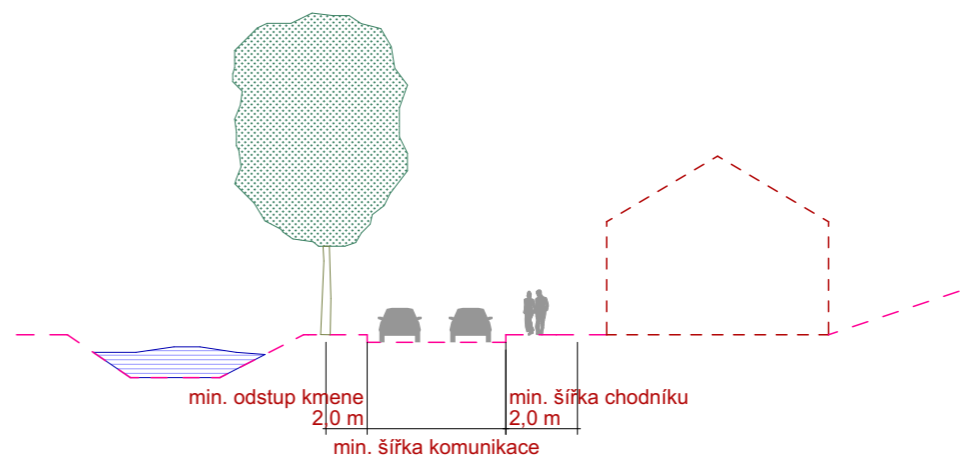
řez obslužnou komunikací Na Návsi - jih návrh
