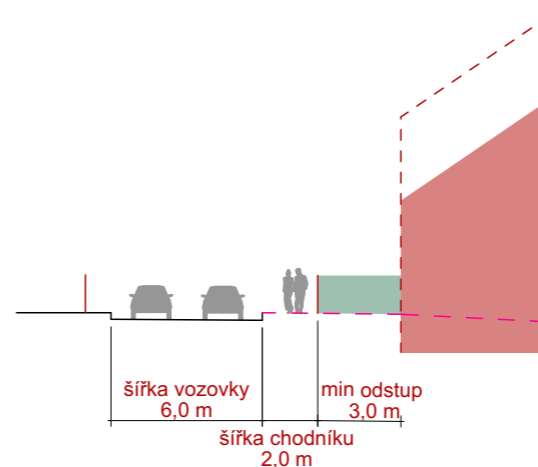
řez silnicí III/10176 - Starobabická návrh
