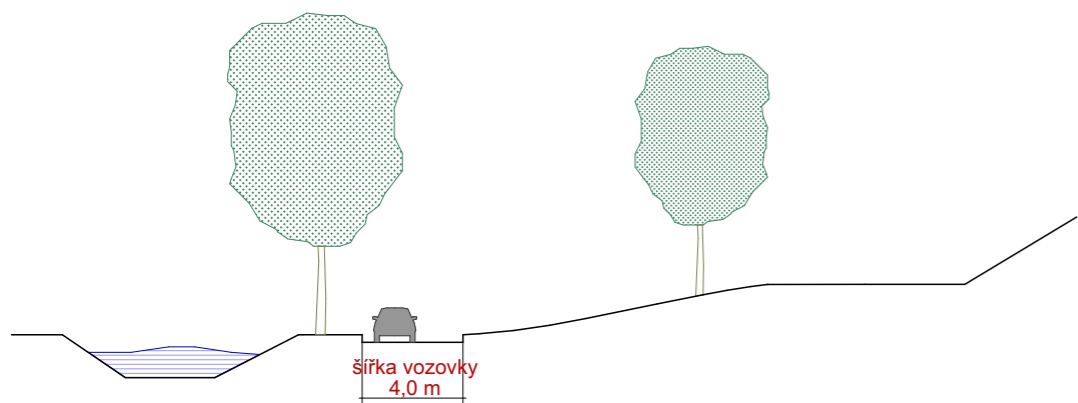
řez obslužnou komunikací Na Návsi - jih stav
